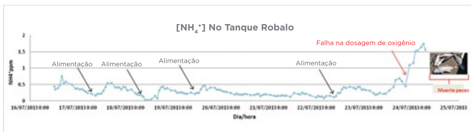
Figura. Exemplo de monitorização da concentração de amônia no tanque robalo
